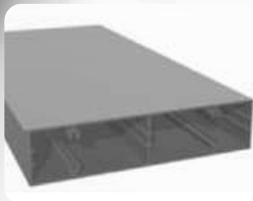
Profil belki/Beam profile/ Strahlprofil W=5,309kg/m (253x55x2,5mm)
